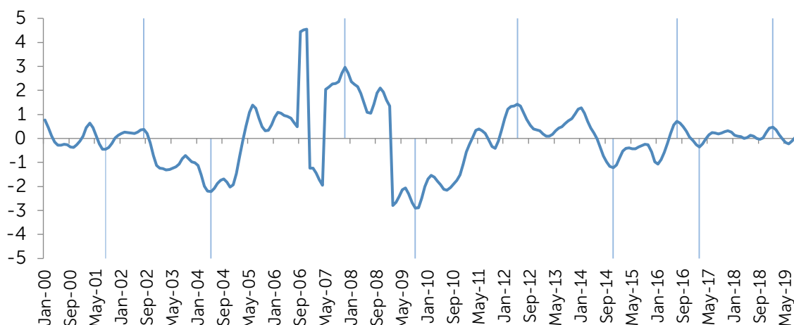
Gráfico 1. Ciclo y puntos de giro del IVAE. 2000 a 2019. 3
