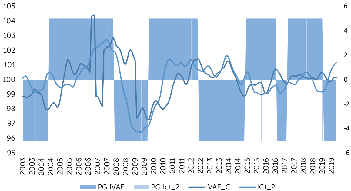
Gráfico 3. Indicador 2 versus ciclo del IVAE y puntos de giro
